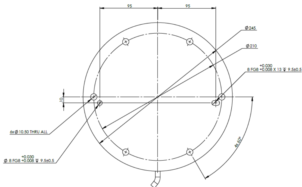
1.1: 機器人底座的底部視圖
