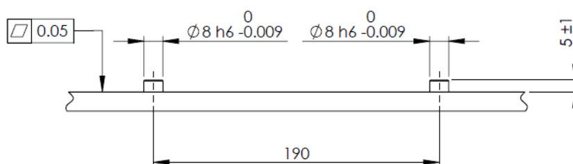
1.2: 機器人底座安裝板
